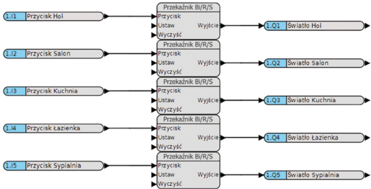
Rys. 7. Schemat podstawowego sterowania oświetleniem całego mieszkania
